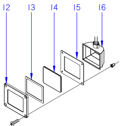
DETALLE DE LAMPARA
