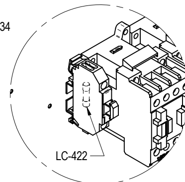
DETTAGLIO A
