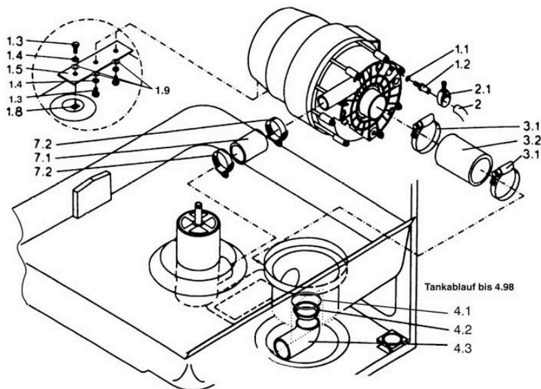
Tankablauf ab Geräte-Nr. 239605
