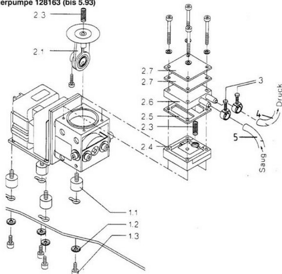
Reiniger Dosierpumpe 128163 (bis 5.93)
